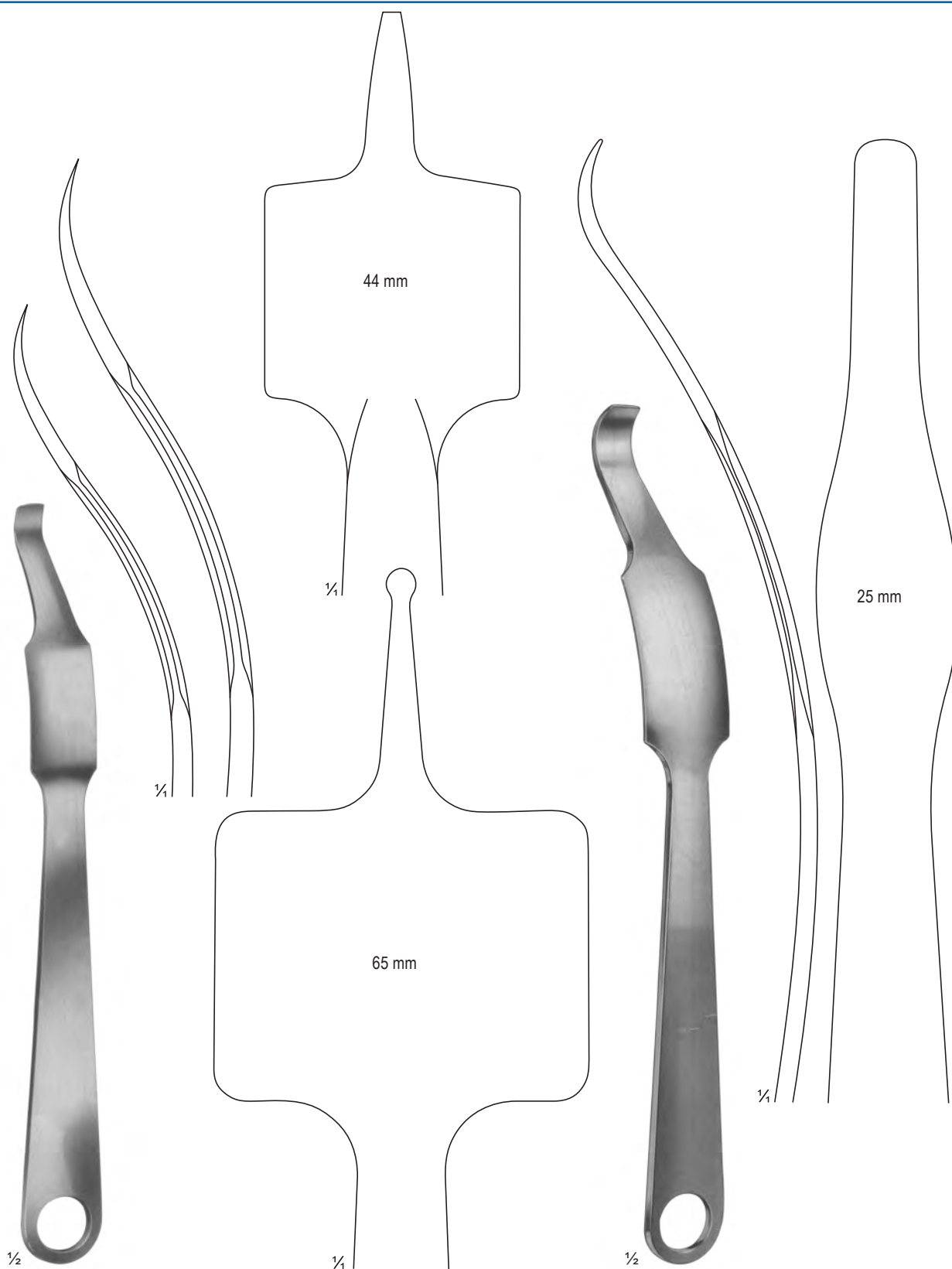
RS-018 - 019 VERBRUGGE-MULLER RS-018 240 mm RS-019 255 mm
