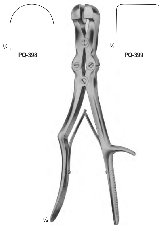
PQ-398 - PQ-399 SAUERDRUCH-CORYLLOS Rib rongeurs to shortn the rib stumps 310 mm
